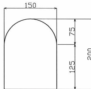
配管用切欠き詳細図
